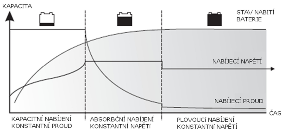
Obr. Dobíjení baterie ve 3 fázích:
